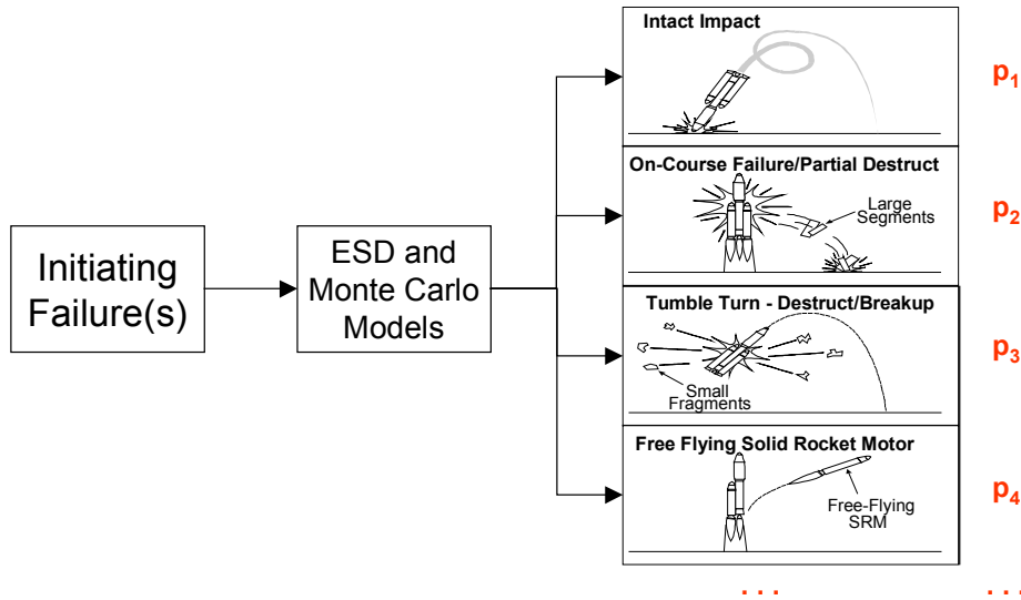
Figure 14-6: Titan IV-SRMU Blast Scenarios
