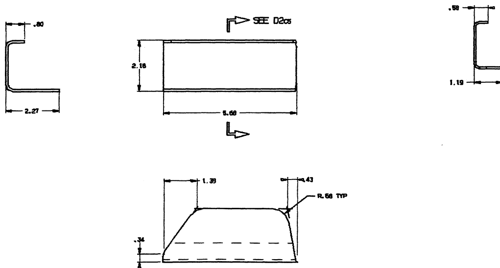
DETAIL-6 SCALE: 1/1
