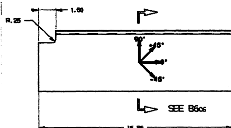
DETAIL-6 SCALE:NONE
