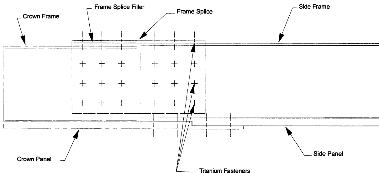
Figure 4-24. Longitudinal Splice
