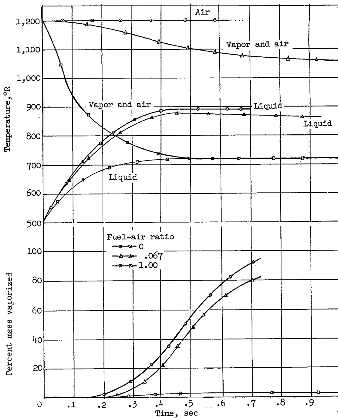
(b) n-hexadecane.
