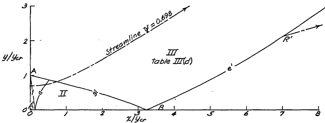
(d) v_B = 40^\circ .
