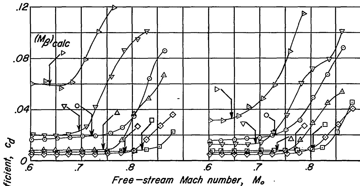
(e) NACA 65, -206.
