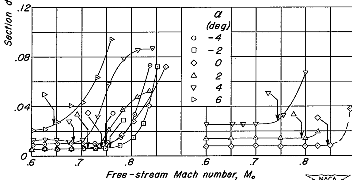
(k) NACA 66,-212.
