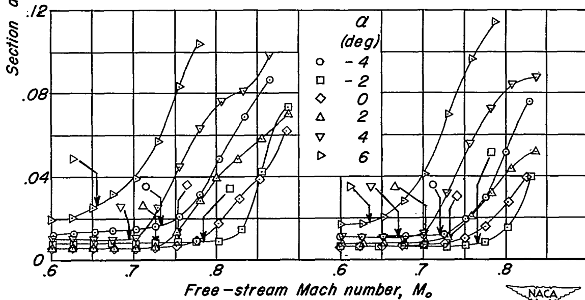
(g) NACA 65, -210
