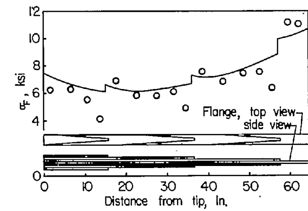
(d) Flange stresses in panel E. P = 7.5 kips.
