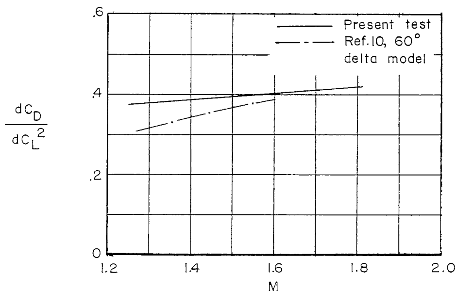
(b) Drag-due-to-lift parameter dC_D/dC_L^2 .
