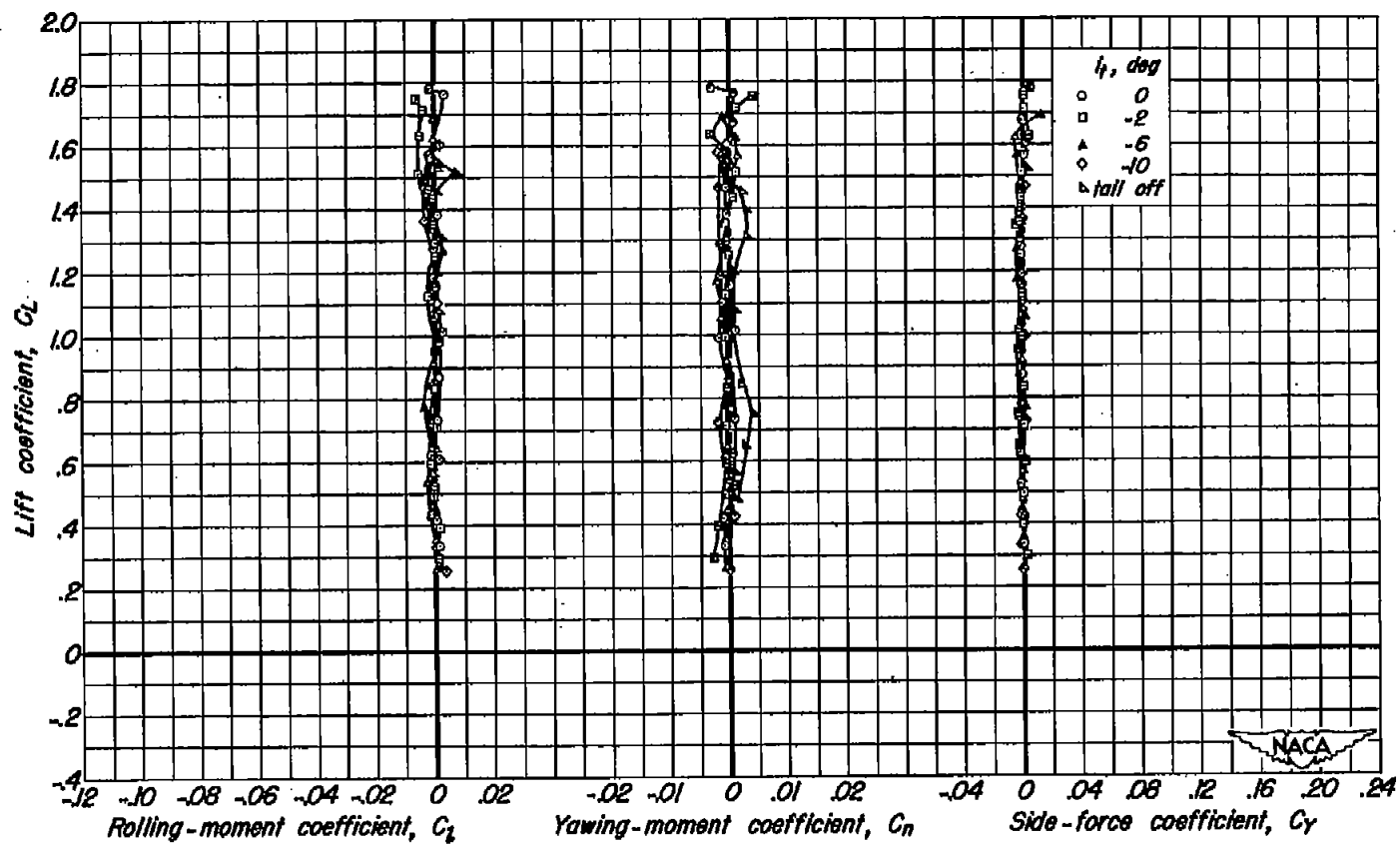
(b) C_L vs C_L , C_n , C_y
