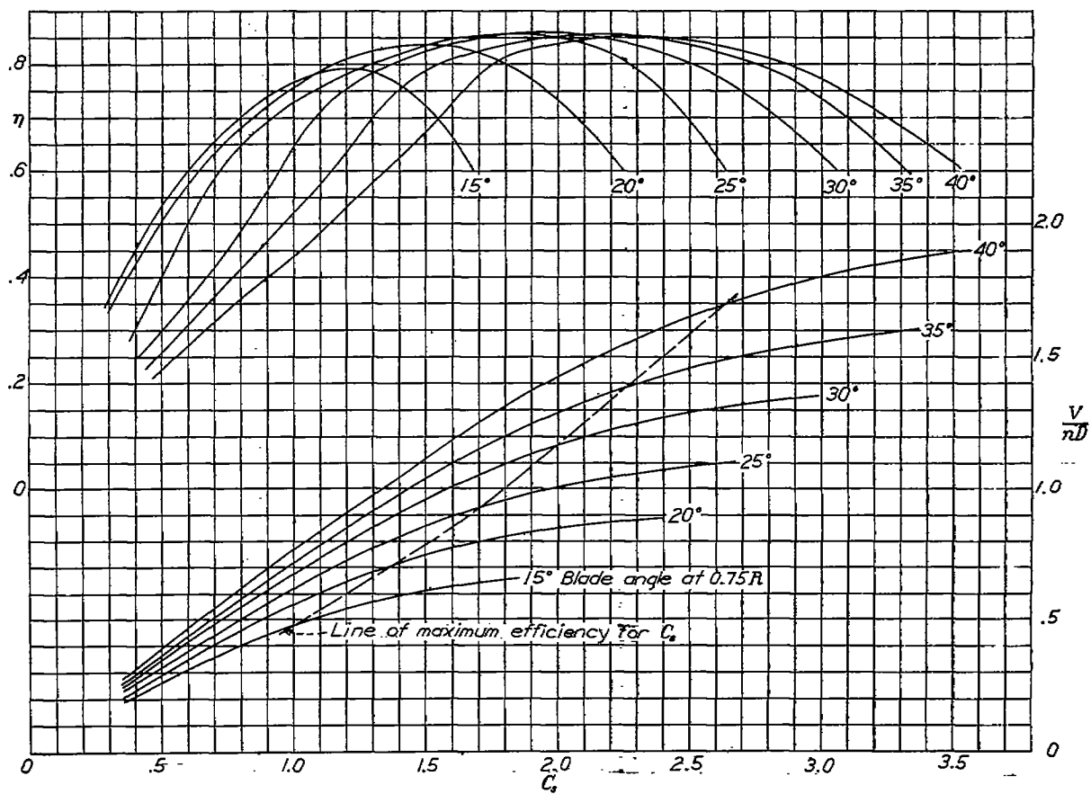
FIGURE 24.—Design chart for propeller 6623-O (N. A. C. A. 2R,00 section).
