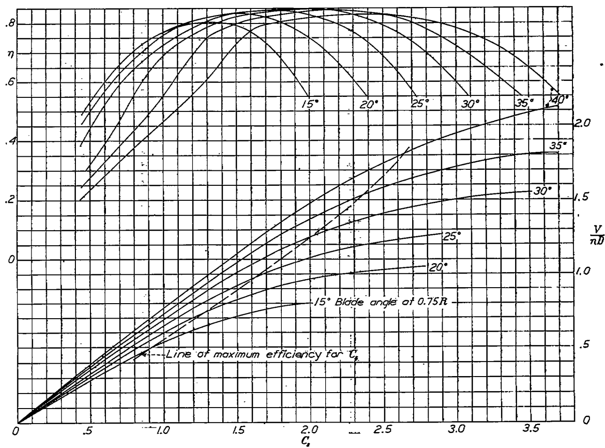
FIGURE 15.—Design chart for propeller 6623-A (N. A. C. A. 4400 section).
