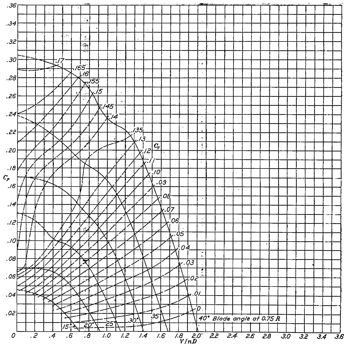
FIGURE 21.—Power-coefficient curves for propeller 6623-O (N. A. C. A. 2R400 section).
