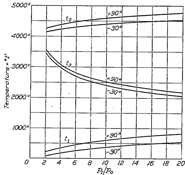
FIG. 2 (Tables 1, 2, 3).—Temperatures
