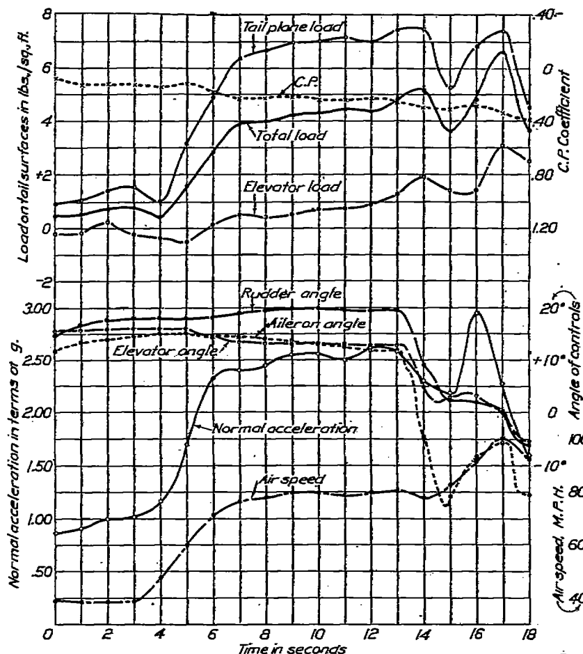
FIG. 22.—Tail spin.
