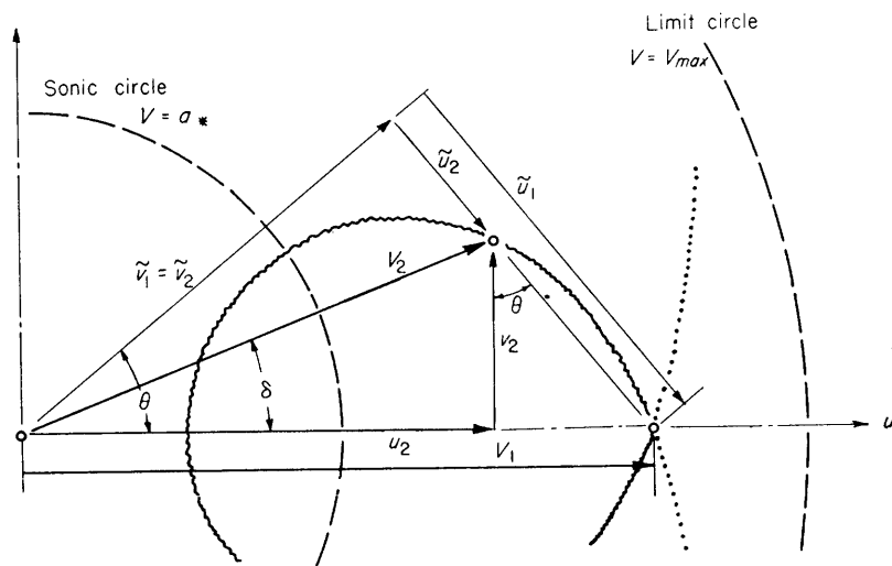
FIGURE 3.—Shock polar.
