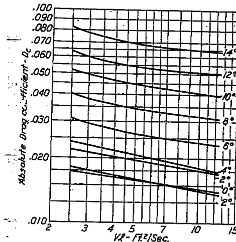
FIG. 6.—Variation of drag coefficient with V_L . Data from B. A. C. A. R. & M. No. 110. R. A. F. 6 Aerofoil.
