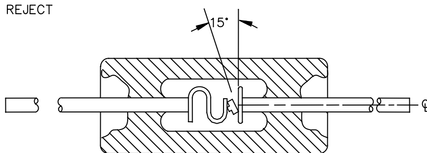
FIGURE 2074-A11. Die alignment .
