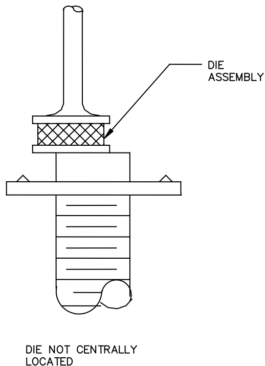
FIGURE 2074–H1. Offset die .
