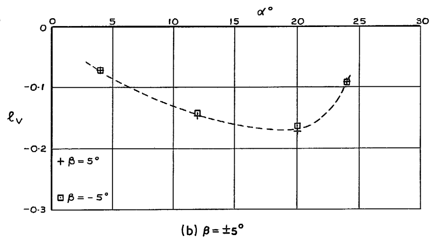
FIG. 6a & b. BAC 221 l_v vs \alpha .
