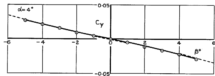
FIG. 8. BAC 221 C_y vs \beta .
