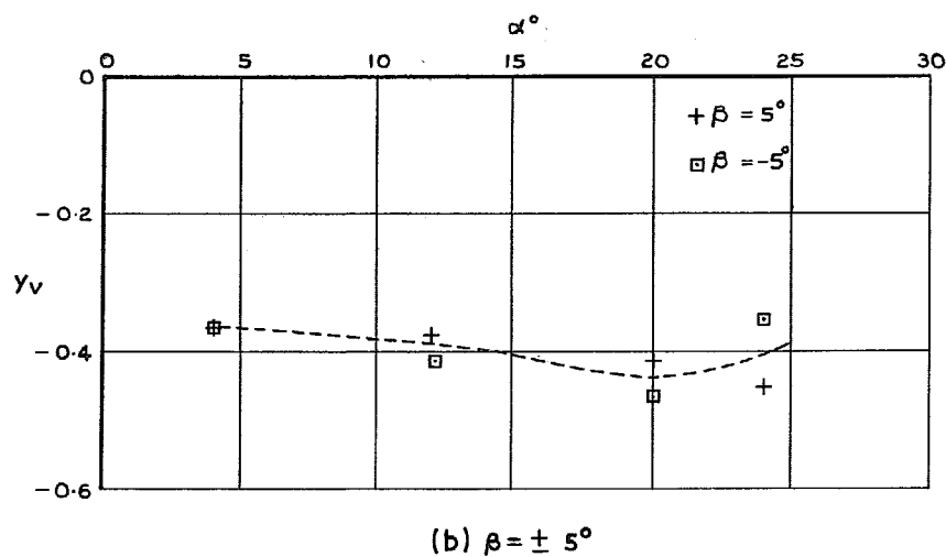
FIG. 5a & b. BAC 221 y_v vs \alpha .
