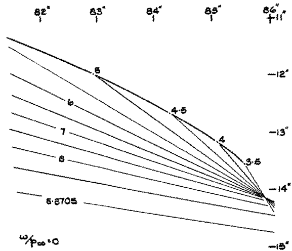
(a) M_N = 1.4 , p_u/p_{\infty} = 0.5
