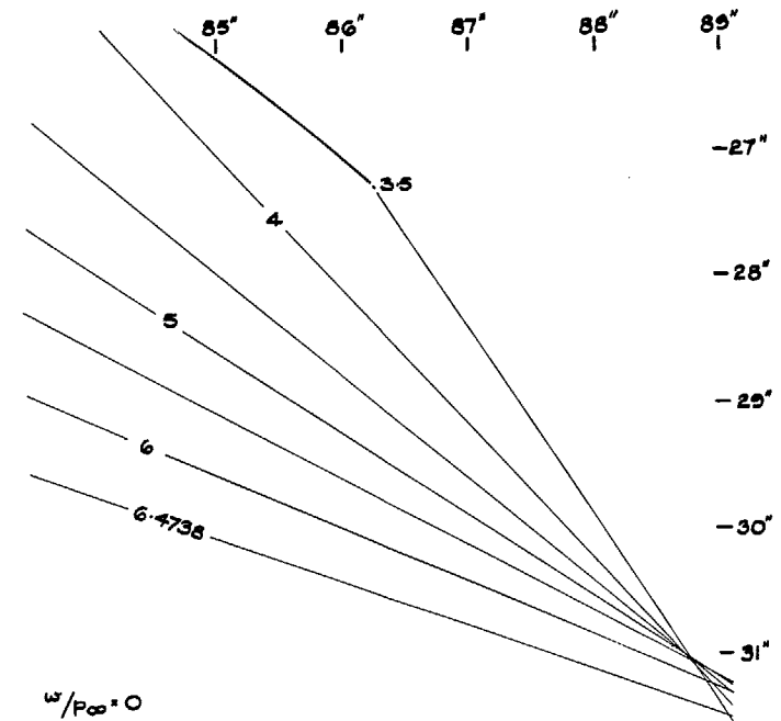
(d) M_N = 2.6 , p_u/p_\infty = 1.0
