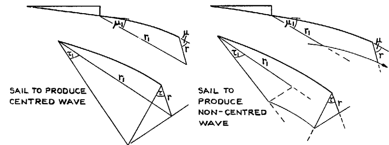
(d) GEOMETRY OF SINGLY CURVED SAILS
