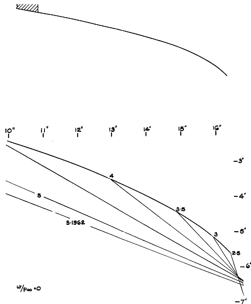
(d) M_N = 2.0 , p_u/p_\infty = 1.0
