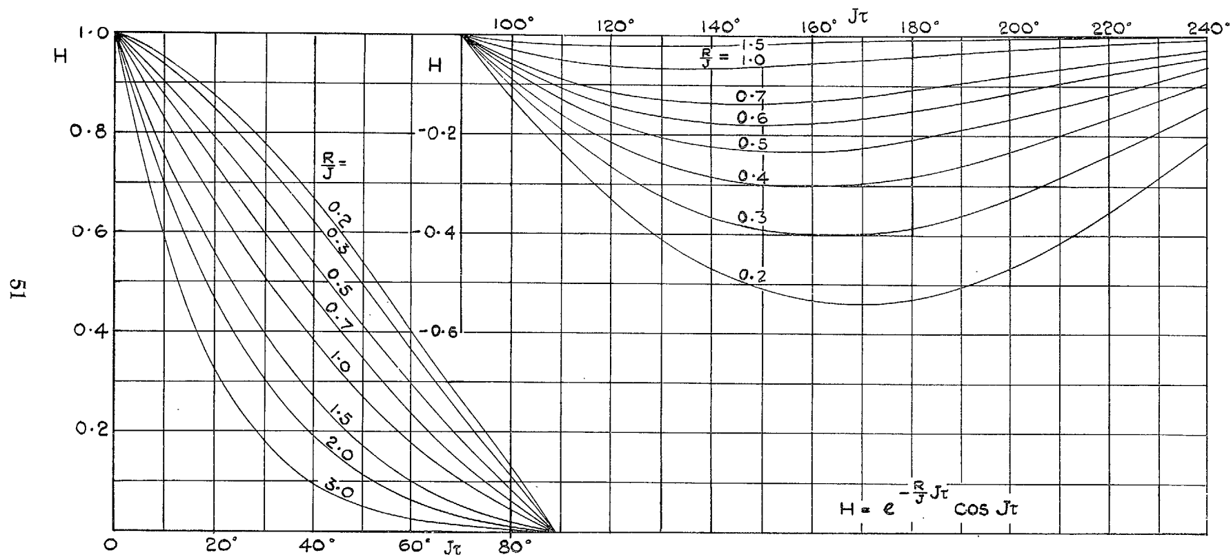
FIG. 5. Function H .
