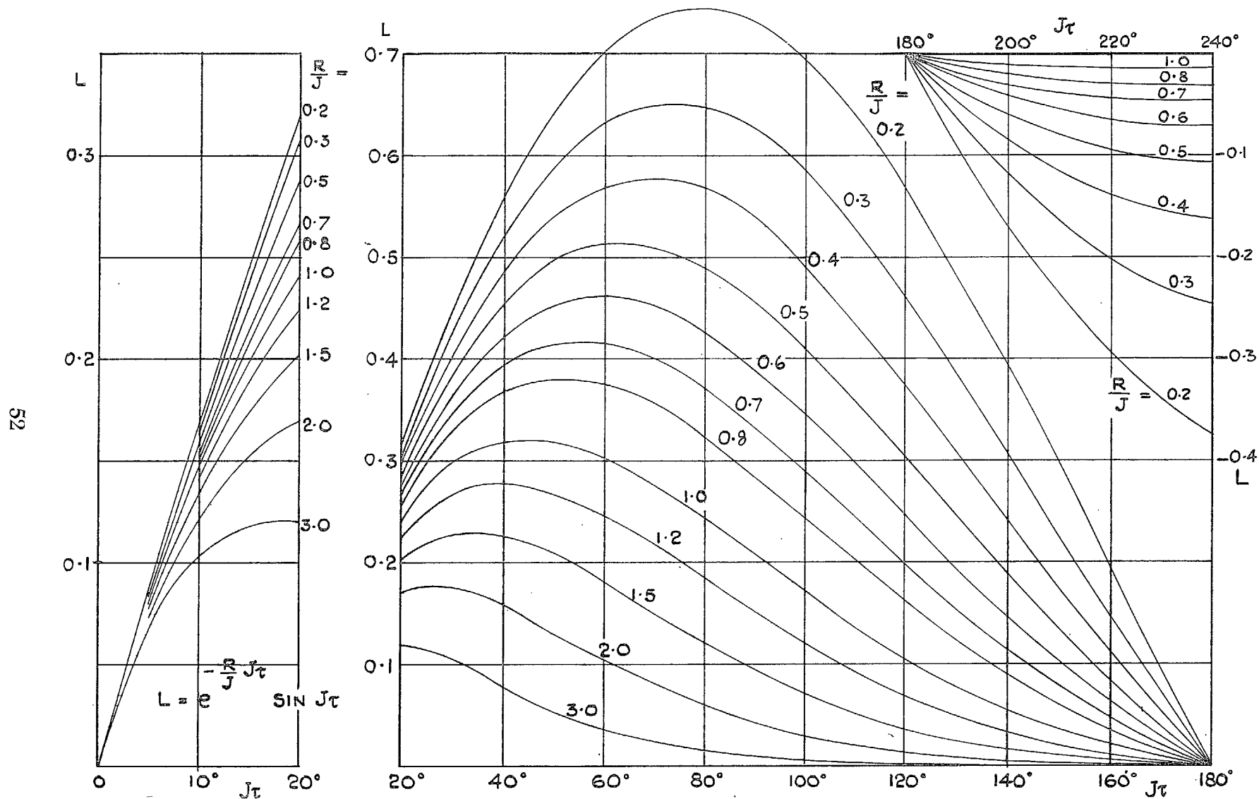
FIG. 6. Function L .
