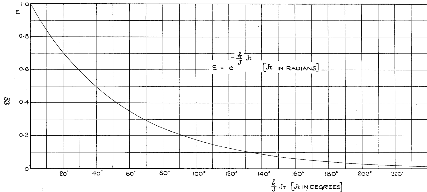
FIG. 7. Function E .
