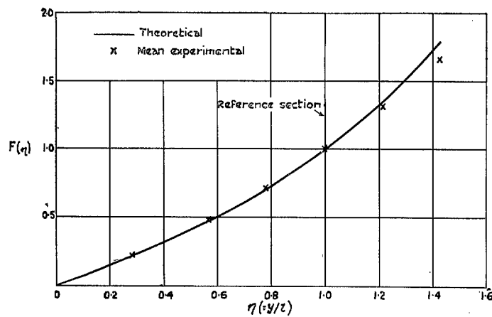
FIG. 7.—Torsional Mode.
