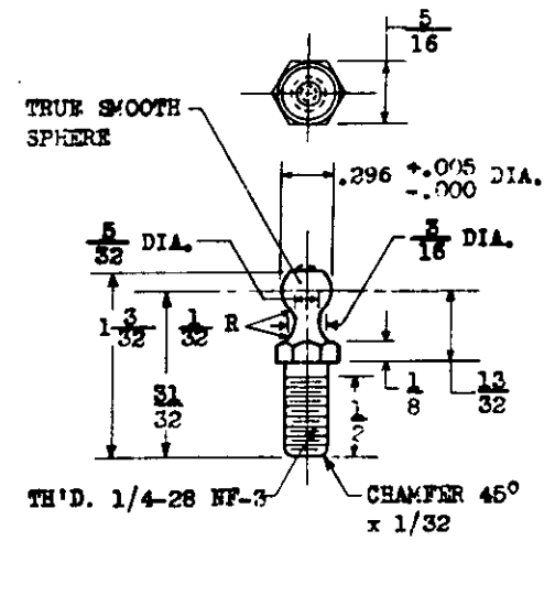
AN276-2 BOLT (NICKEL OR MOLY. STEEL)
