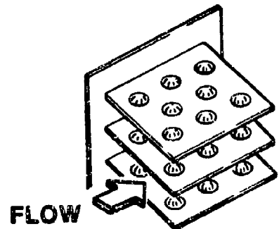
(D) DIMPLED FIN
