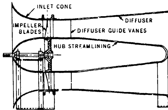
(D) VANE-AXIAL WITH DIFFUSER (Courtesy of Buffalo Forge Co.)
