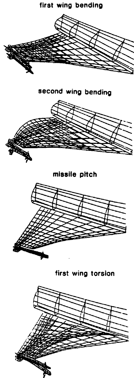
Fig.: 3 Vibration Modes
