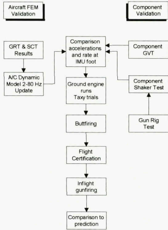
Fig.: 40 Modal Validation
