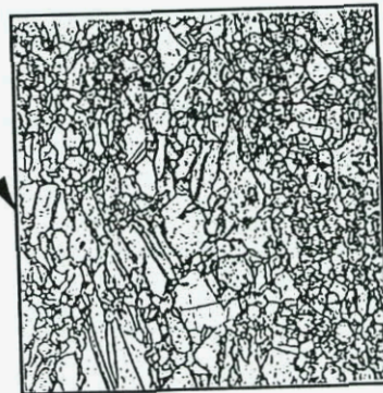
8-9 ASTM recristallisé
