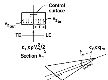
Fig. 29. Vortex action point concept; Lan.
