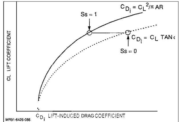
Fig. 56 S_s Parameter Definition
