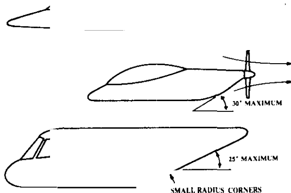
Fig. 15 Longitudinal contour guidelines
