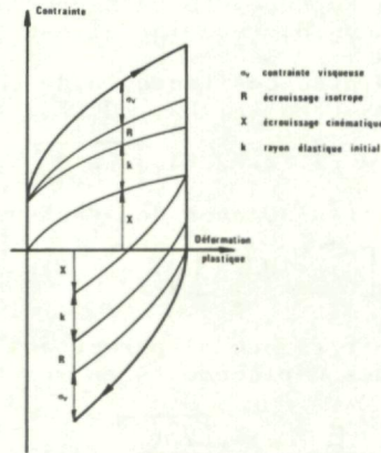
Figure 5 : Phénomènes viscoplastiques
