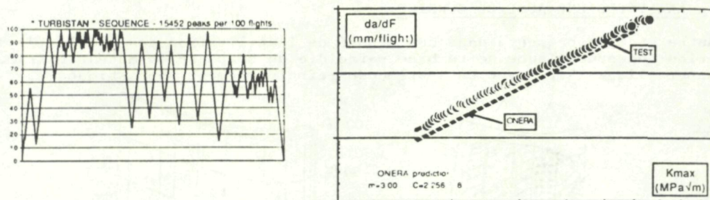
Figure 7 : Essais sur INCO718 à 450° C sur séquence TURBISTAN
