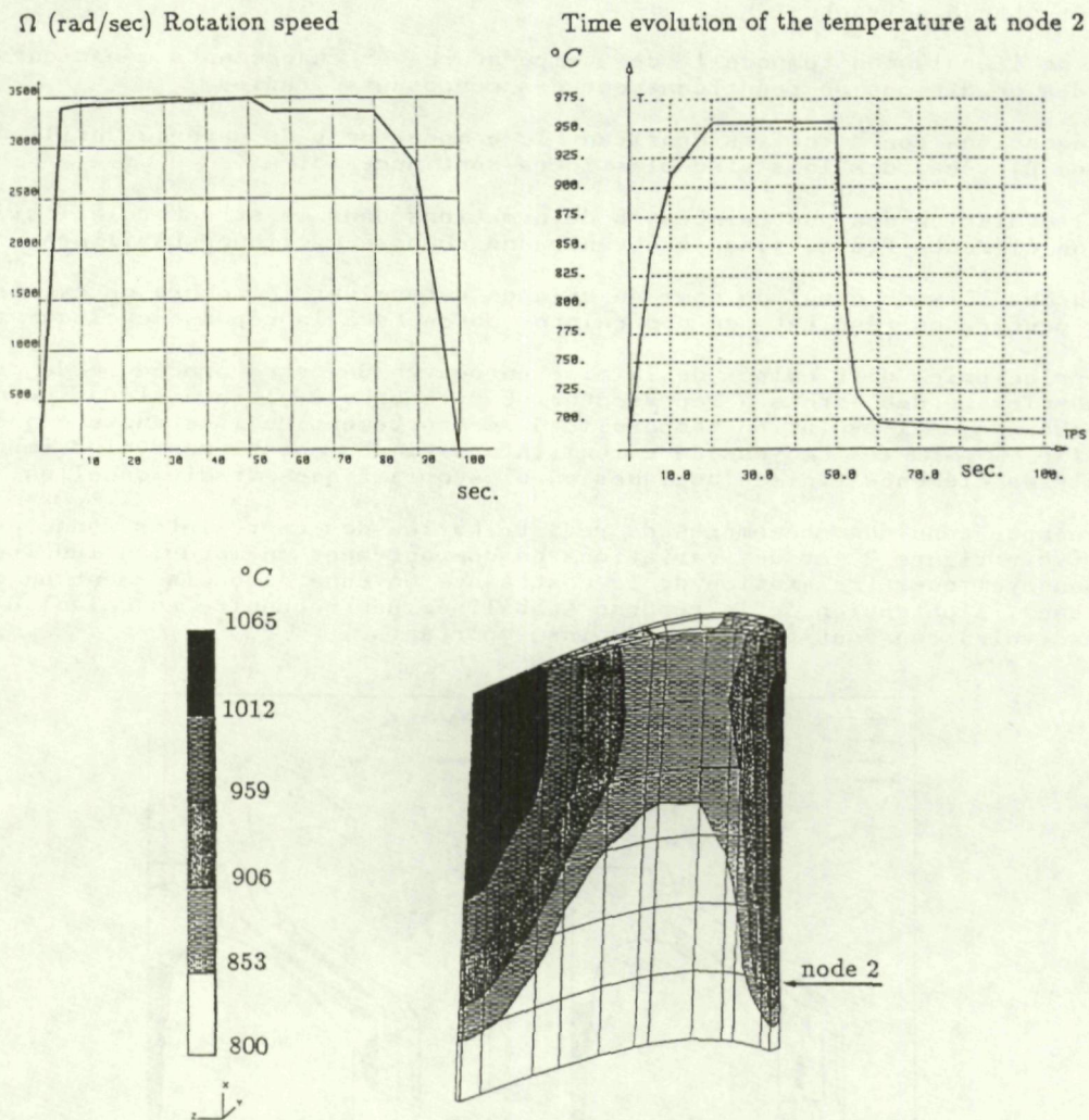
Figure 9: Cycle de chargement thermique et mécanique de l'aube
