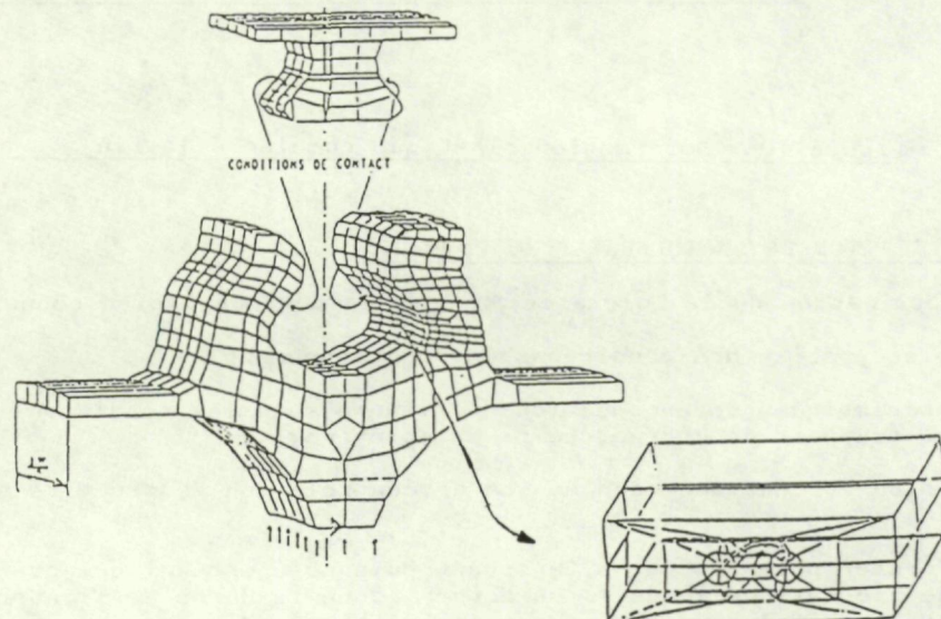
Figure 12 : Exemple d'étude en fissuration d'un fond d'alvéole de disque de compresseur avec le détail des éléments variables contenant la fissure
