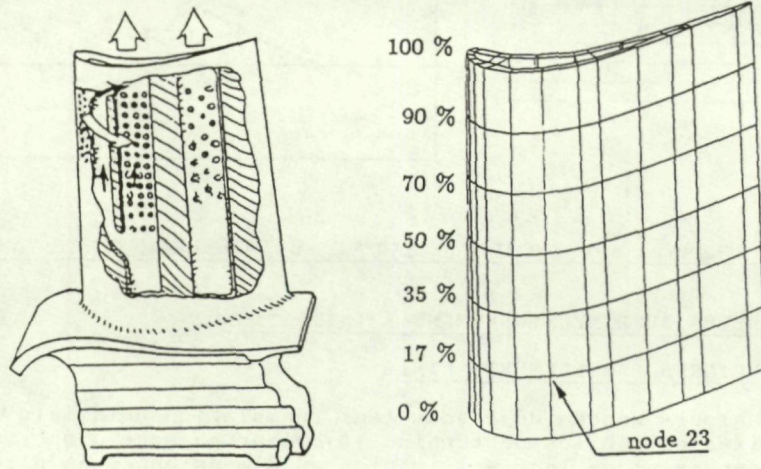
Figure 8 : Géométrie et maillage de la pale
