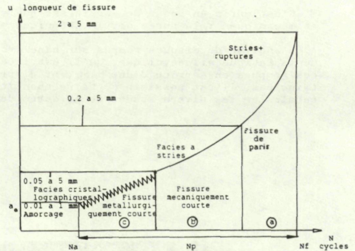
Figure 4 : Stades de la durée de vie en fissuration par fatigue
