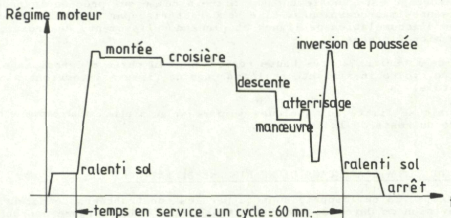
Figure 1 : Cycle de vol typique pour turboréacteur civil
