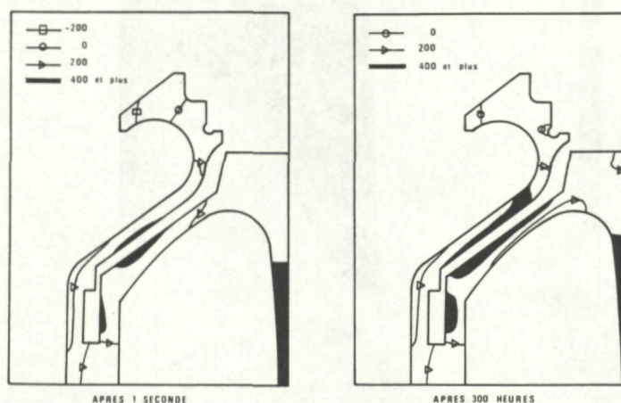
Figure 7 : Redistribution des contraintes circonférentielles sur un rotor de turbine suite à un temps de maintien à haute température
