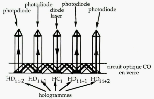
Figure 5 Connecteur optique de fond de panier pour baie électronique (en haut, perspective ; en bas, coupe).
