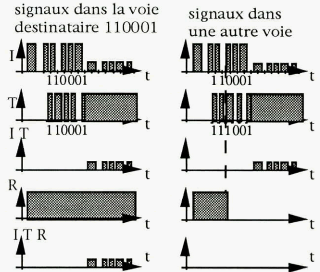
Figure 7 Principe de la logique de reconnaissance d'adresse par voie optique. I = lumière incidente. T = transmission du modulateur électro-optique. R = réflectivité du bistable.
