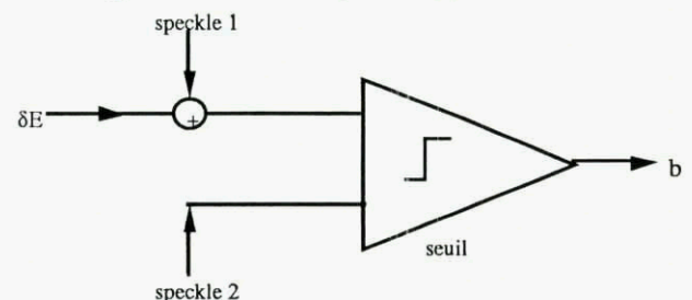
Figure 9. Génération de la loi de probabilité de l'équation (3) à l'aide de deux échantillons de speckle.
