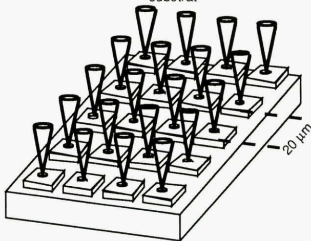
Figure 2. Matrice de lasers à cavité verticale.
