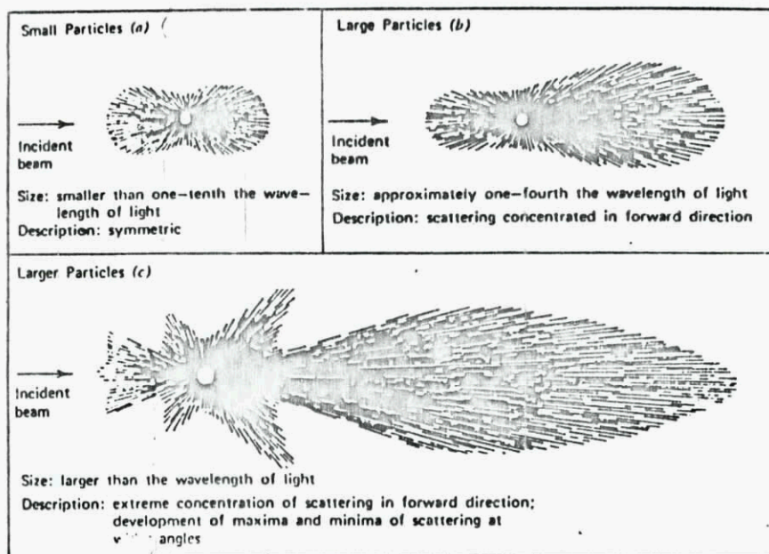
Fig. 1 Répartition angulaire de l'intensité diffusée par des particules de trois tailles : (a) petites particules, (b) particules moyennes, (c) grosses particules [2]
