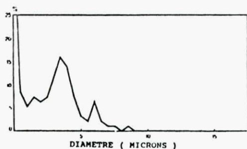
Figure 2: Répartition granulométrique des produits condensés récupérés dans un jet de propulseur analysés par microscopie électronique et spectrométrie X. (SNPE-France)
