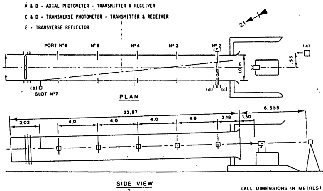
Figure 12: Tunnel à fumée R7 du Royaume Uni (RO)
