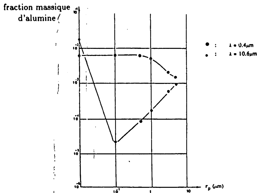
Figure 10: Quantité maximale d'alumine (fraction massique) dans les produits de combustion pour les spécifications suivantes : diamètre du nuage : 1 m, dilution : 0.05, transmission : 95 %.
