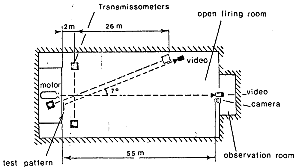
Figure 15: Tir en jet libre. "Banc opacimétrique" SNPE (France)
