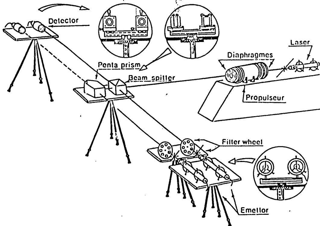
Figure 16: Tir en jet libre. Transmission à 0.63 μm
