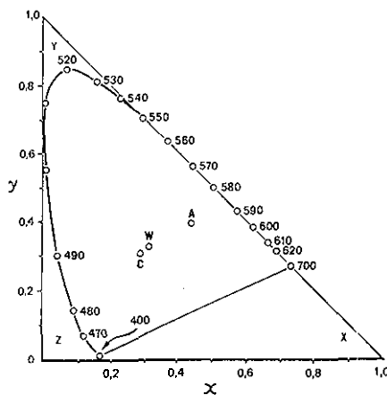
Figure 5 : Triangle des couleurs CIE 1931
