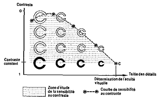
Figure 7 : Acuité visuelle et Fonction de Sensibilité au contraste.
