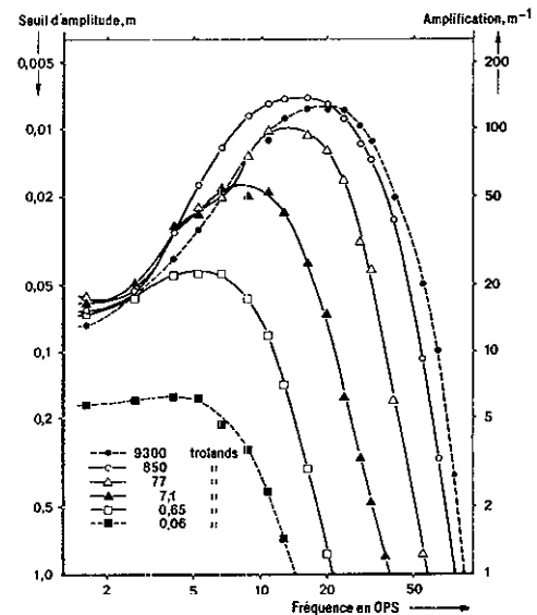
Figure 9 : Sensibilité temporelle (d'après Kelly 1961)
