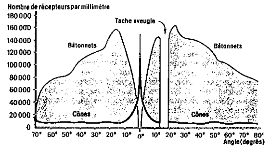
Figure 3 : Densité des photorécepteurs avec l'excentricité
