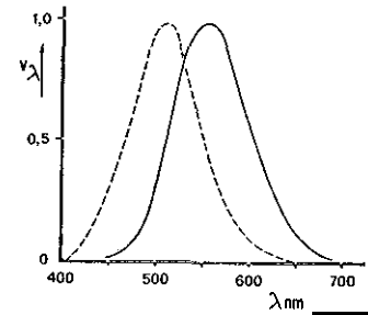
Figure 4. Courbes d'efficacité lumineuse relative
