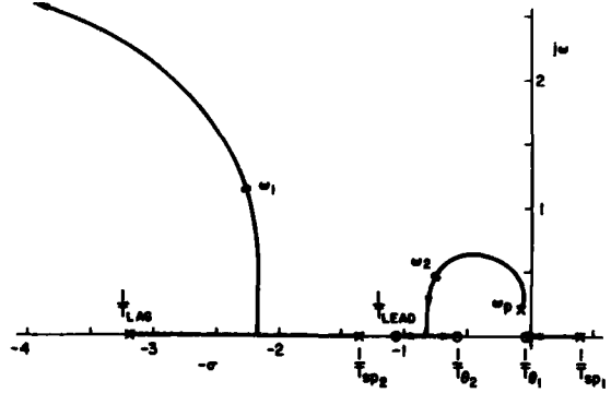
b) q - \delta_p Feedback
