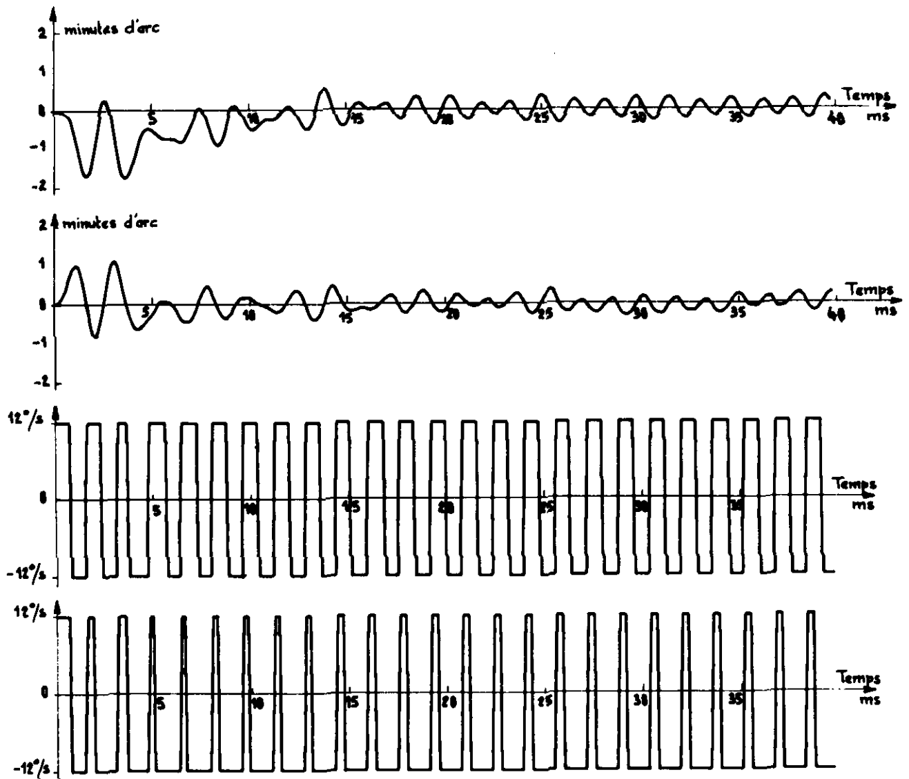
Figure 23 - Simulation de la réponse d'un gyro GAM3 à un échelon de vitesse angulaire
