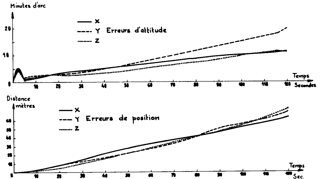
Figure 25 - Résultats obtenus en simulation
