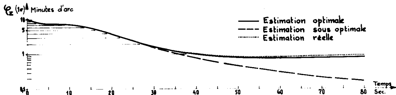
— Figure 29 — Simulation d'alignement
