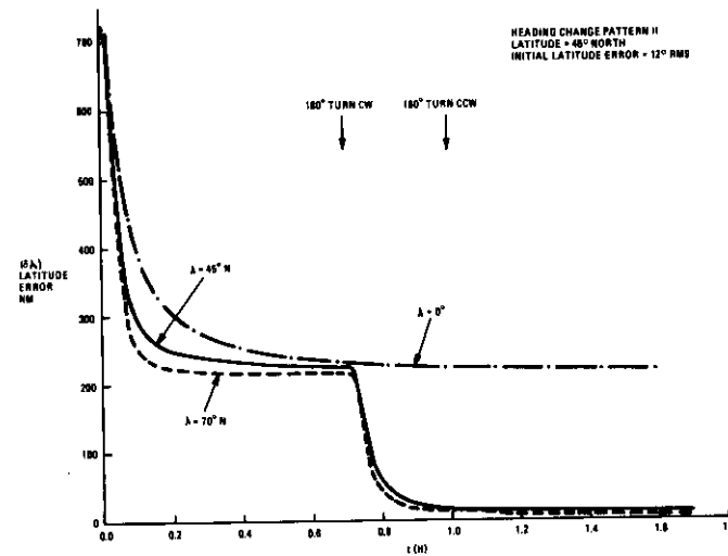
Figure 25. Effect of Operating Latitude on Latitude Error
