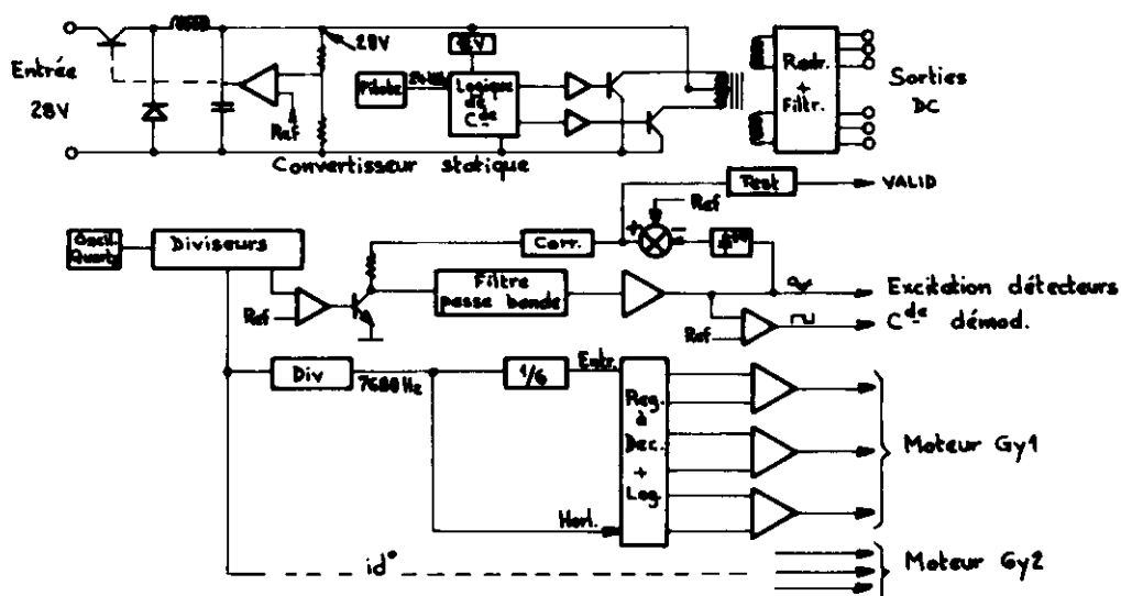
Figure 12 – Fonctions générales
