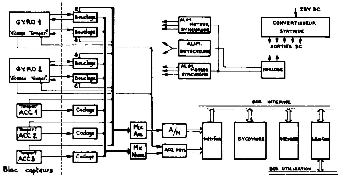
Figure 7 : Diagramme Fonctionnel SIL3
