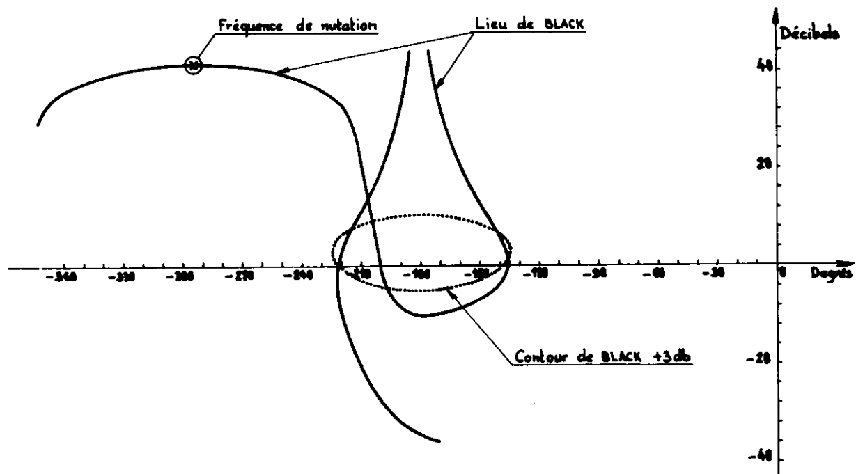
Figure 14 - Analyse d'une boucle gyromètre numérique [Lieu de BLACK]
