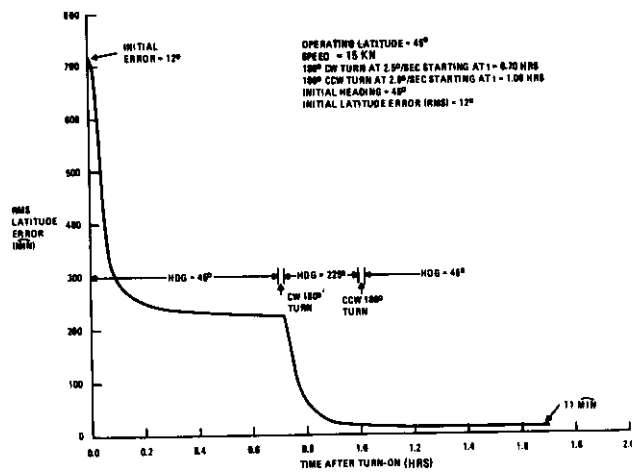
Figure 23. RMS Latitude Error At-Sea Performance
