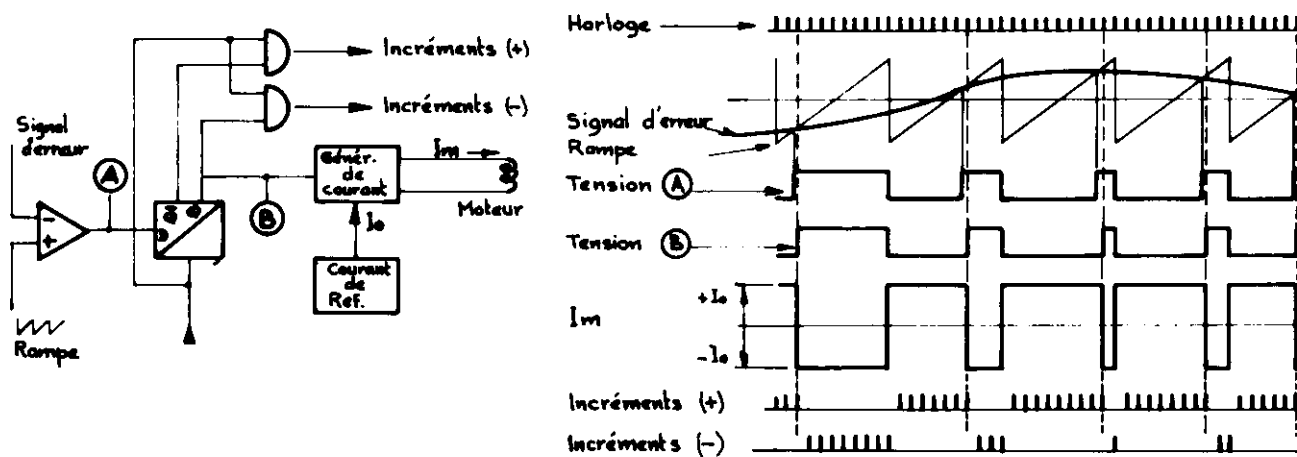
Figure 13 - Principe de bouclage en modulation de longueur
