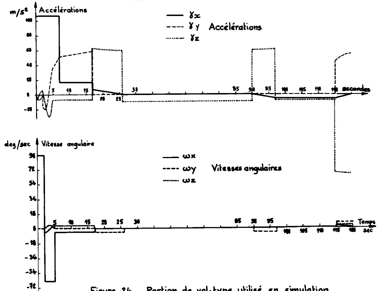
Figure 24 - Portion de vol-type utilisé en simulation
