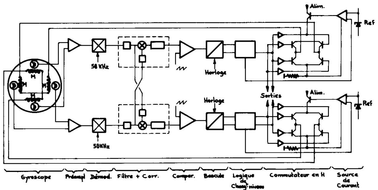
Figure 15 - Boucle gyromètre . Schéma de principe
