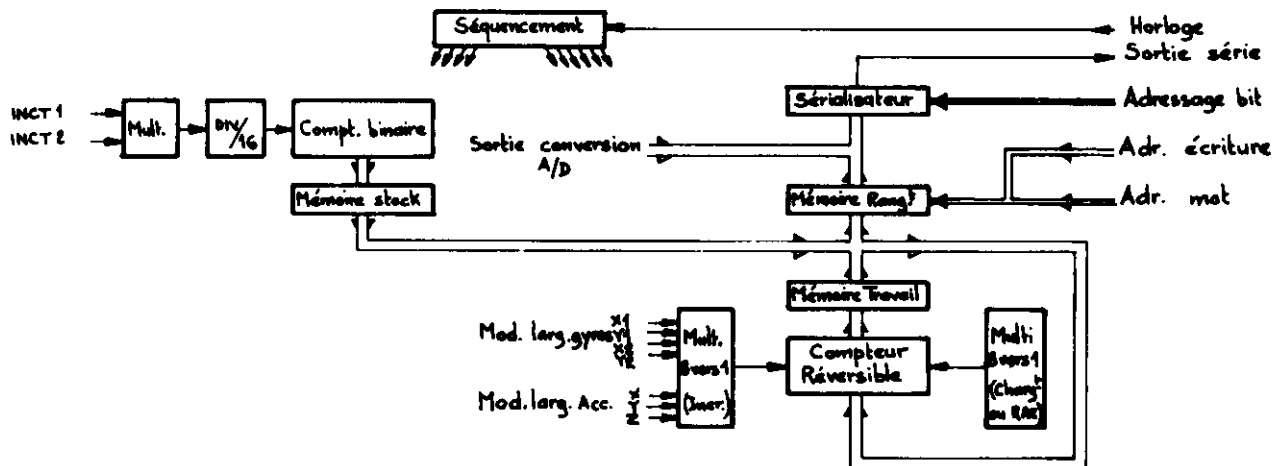
Figure 17 - Logique de comptage et transmission série
