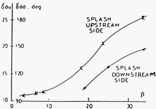
FIG. 14. INITIAL EJECTION ANGLES ( t=0 )
