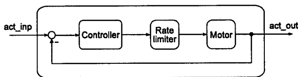
Fig 1 Actuator
