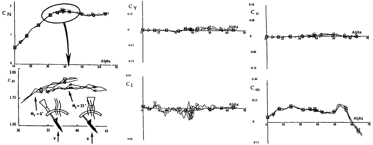
Fig 3.62 - BWLHVST Configuration - slow AOA sweeps - Repeatability tests ▲ 209 : \Theta_2 = 0^\circ ○ 203 : \Theta_2 = 25^\circ ▼ 500 : \Theta_2 = 0^\circ ◊ 211 : \Theta_2 = 25^\circ ◇ 709 : \Theta_2 = 0^\circ ◐ 711 : \Theta_2 = 25^\circ
