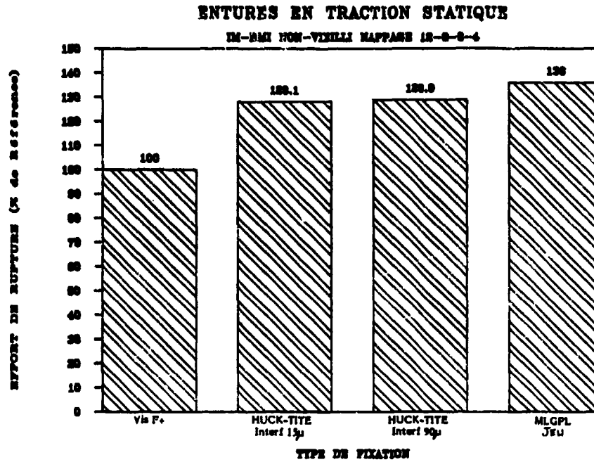
Planche 9 - Essais en traction sur entures IM-BMI.
