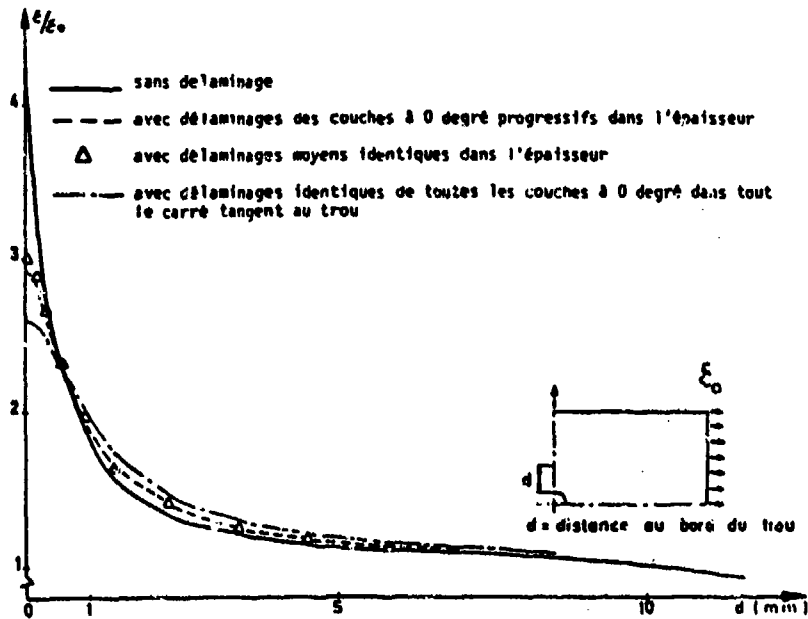
Planche 13 - Schématisation des délamination au bord d'un trou en traction.
