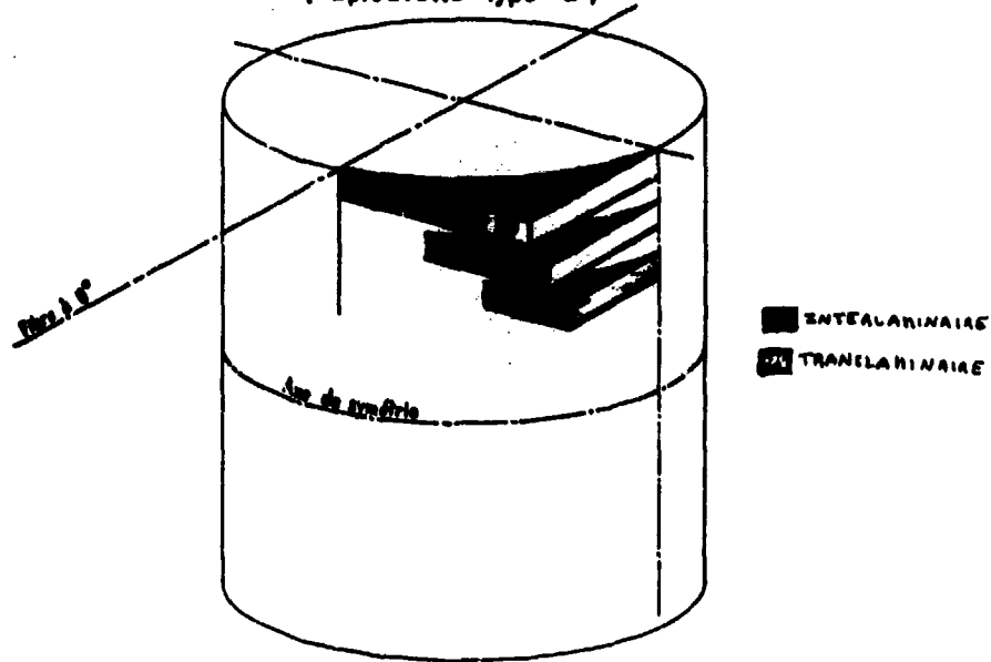
Planche 13 - Schématisation des délamination au bord d'un trou en traction.
