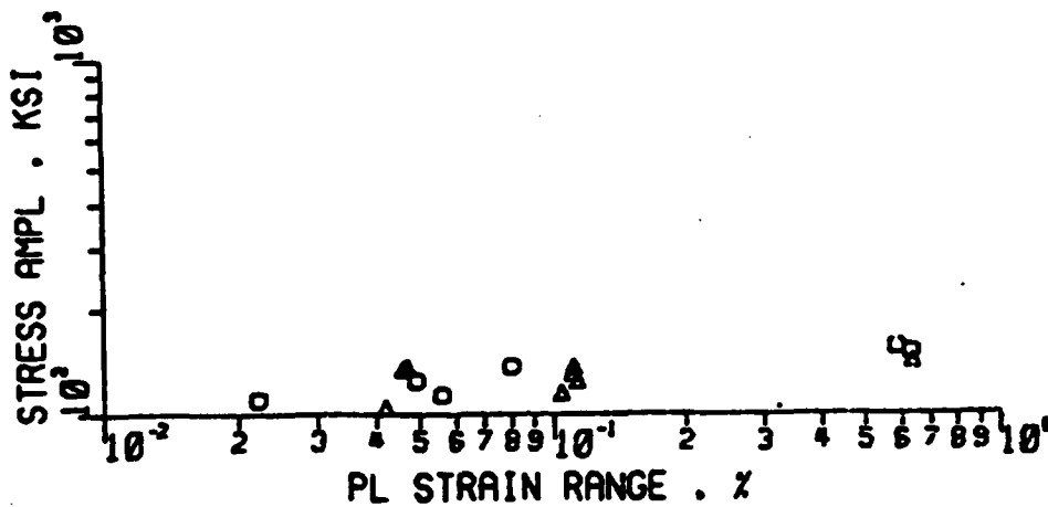
(e) o 010 n' = 0.092; Δ 011 n' = 0.052.
