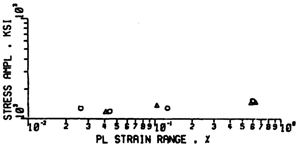
(d) o 0.000 n' = 0.069 ; Δ 0.001 n' = 0.070 .
