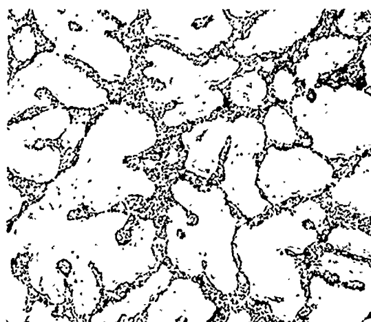
(d) Ti-2.7Be-5Zr (8992) Heat 24107
