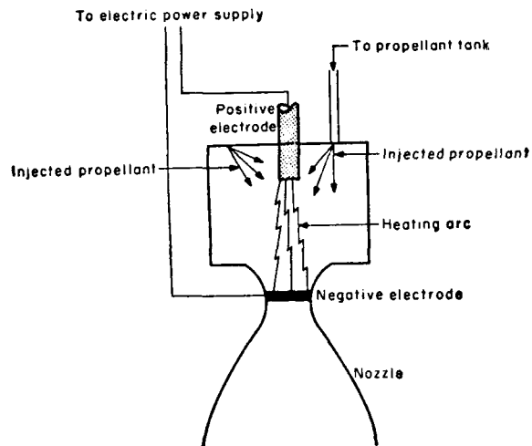
Fig.6-Plasma jet
