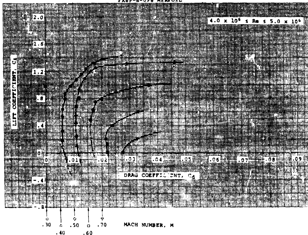
FX69-H-098 AIRFOIL
