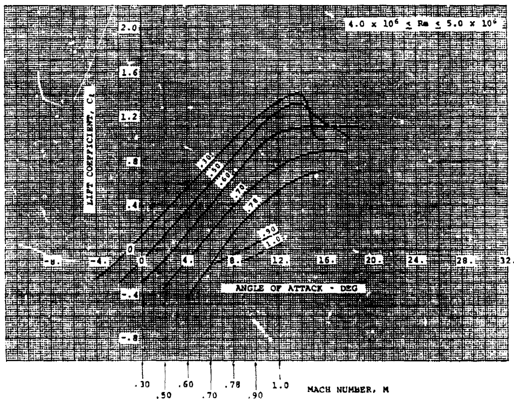
FX69-H-098 AIRFOIL
