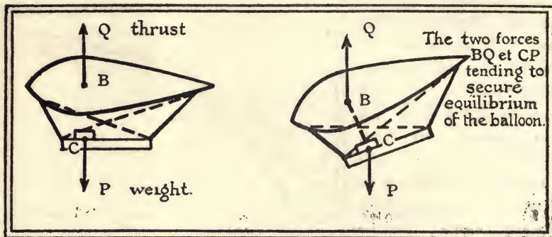
FIG. 9. Longitudinal stability
