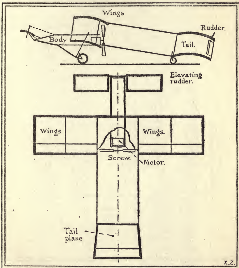
FIG. 69. The Voisin aeroplane (Delagrangé type)
